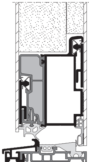
2dílný práh po obvodu s bezfalcovým křídlem
