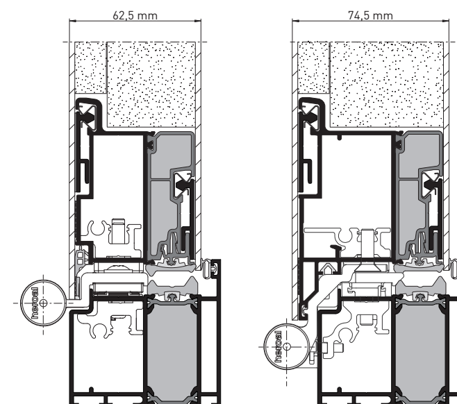
heroal D 72 PF EM bs, Znáznornění průřezu
