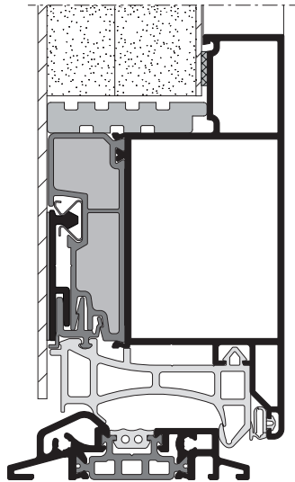
Sešroubovaný práh s falcovým křídlem
