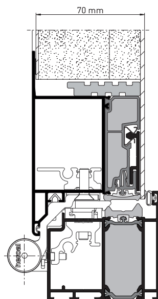
heroal D 72 PF EM 70 mm, Znáznornění průřezu
