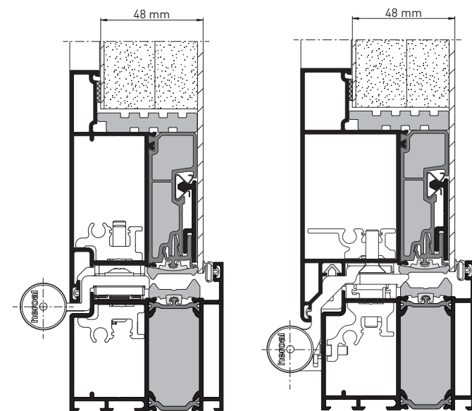
heroal D 72 PF EM es, Znáznornění průřezu
