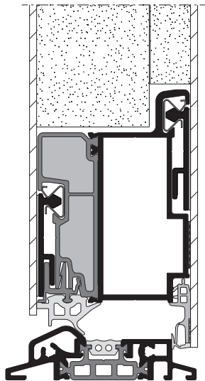
Sešroubovaný práh s bezfalcovým křídlem
