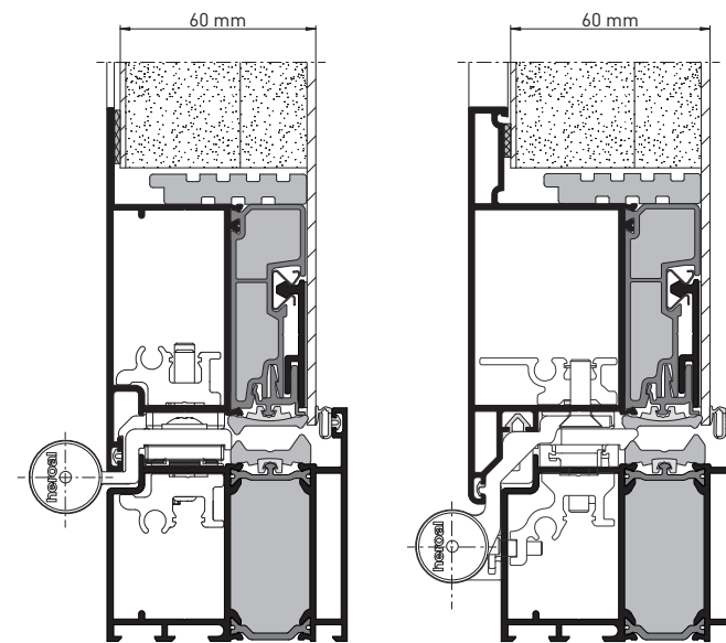
heroal D 72 PF EM es 60 mm, Znáznornění průřezu
