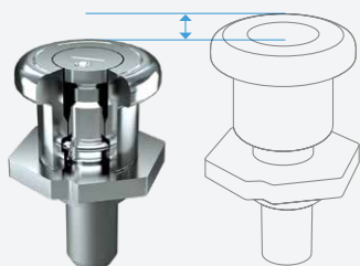
Komfortpilzbolzen mit integrierter Höhenverstellung
